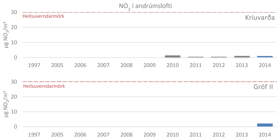
Mynd 4.14: Meðalstyrkur \text{NO}_2 að Kríuvörðu og Gröf II ásamt heilsuverndarmörkum
