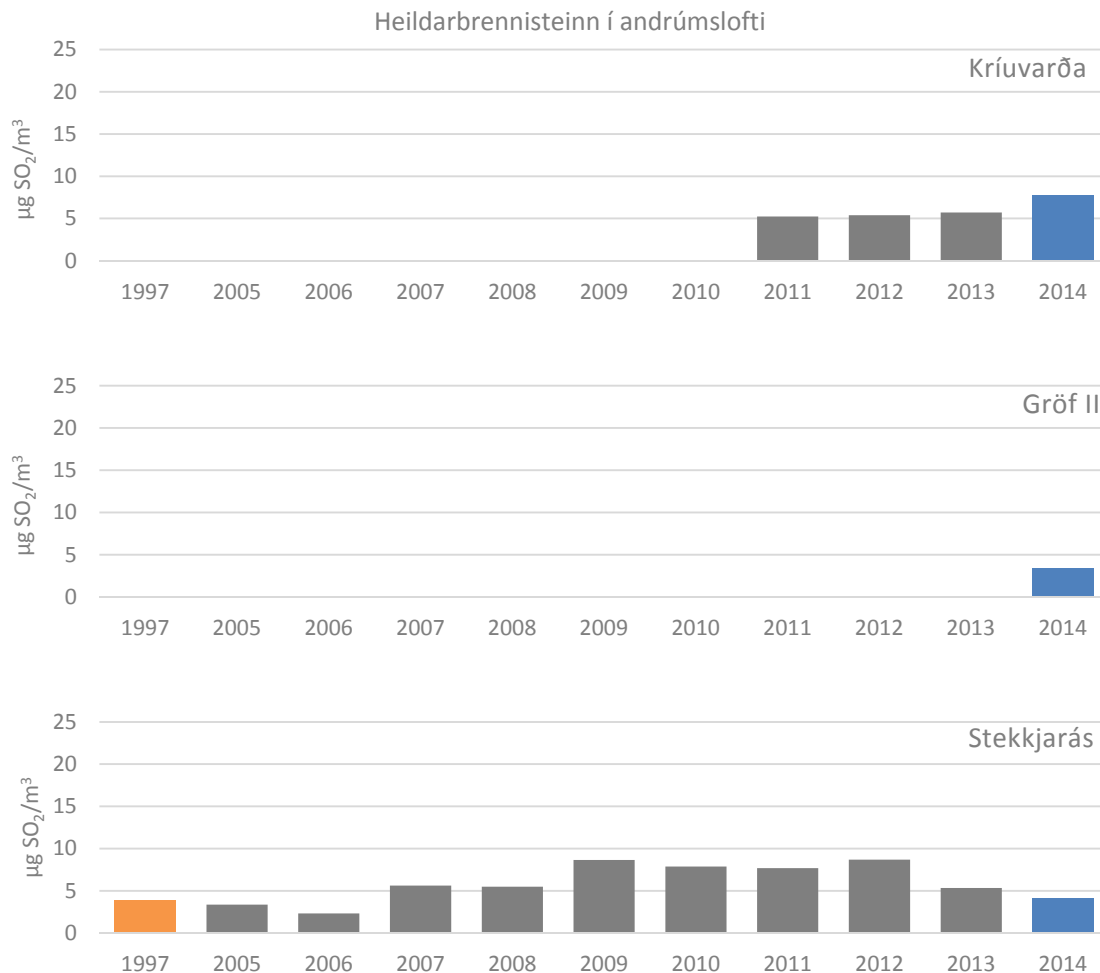
Mynd 4.8: Meðalstyrkur heildarbrennisteins að Kríuvörðu, Gröf II og Stekkjarási yfir vöktunartímabilið (apríl - október en apríl - september 2014).
