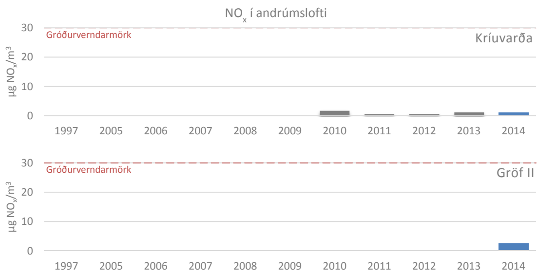
Mynd 4.15: Meðalstyrkur \text{NO}_x að Kríuvörðu og Gröf II ásamt gróðurverndarmörkum
