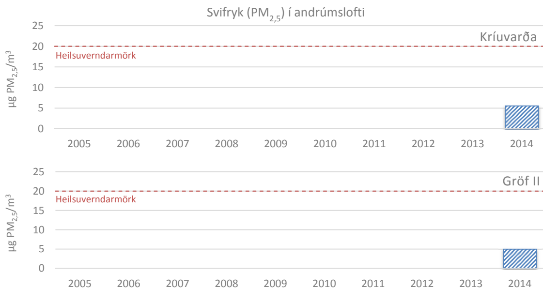
Mynd 4.18: Meðalstyrkur svifryks ( PM_{2,5} ) í andrúmslofti að Kríuvörðu og Gröf II ásamt heilsuverndarmörkum PM_{2,5} sem gilda utan þýnningarsvæðis
