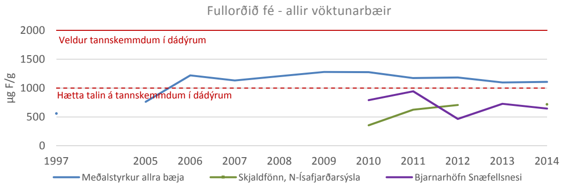
Mynd 10.7: Meðalstyrkur flúors í kjálkabeinum fullorðins fjár árin 2005 - 2014, allir vöktunarbærir í Hvalfirði teknir saman, og viðmiðunarsýni frá 1997
