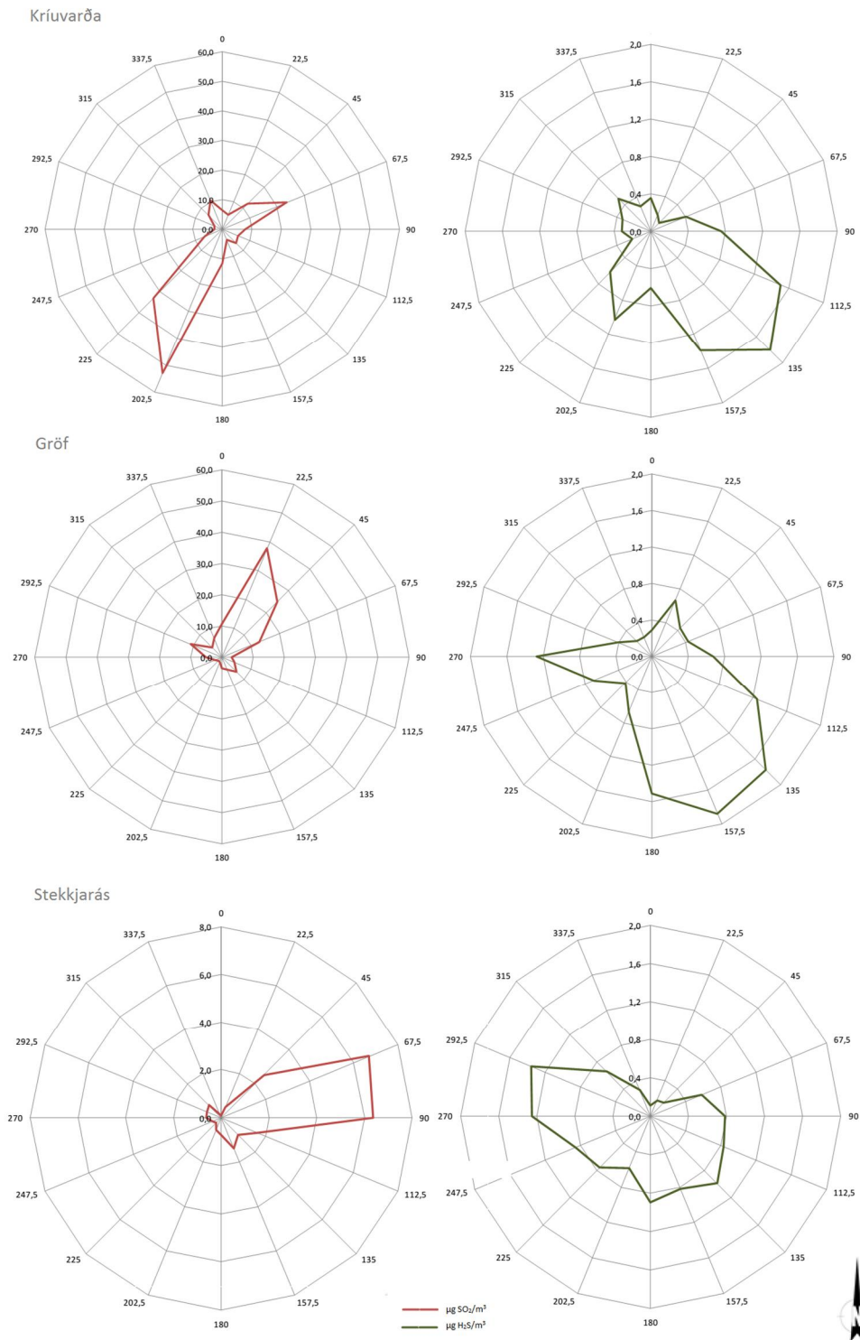
Mynd 4.13: Styrkur SO 2 (rauðar línur, µg SO 2 /m 3 ) og H 2 S (grænar línur, µg H 2 S/m 3 ) í mældum vindáttum árið 2014 að Kriuvörðu, Gröf II og Stekkjarási. Gröfin eru ekki í sama kvarða
