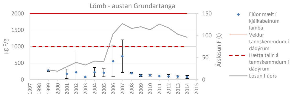
Mynd VI. 2: Meðalstyrkur flúors í lömbum austan Grundartanga ásamt 95% öryggisbilum og heildarlosun flúors í tonnum frá álverinu 1997 – 2014
