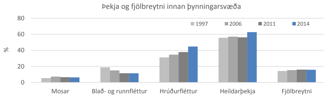
Mynd 7.3: Meðalþekja mosa, blað- og runnfléttna, hróðurfléttna auk meðalheildarþekju og meðal tegundafjölda í öllum fóstum reitum, innan þýningarsvæða, sem metnir voru 2014
