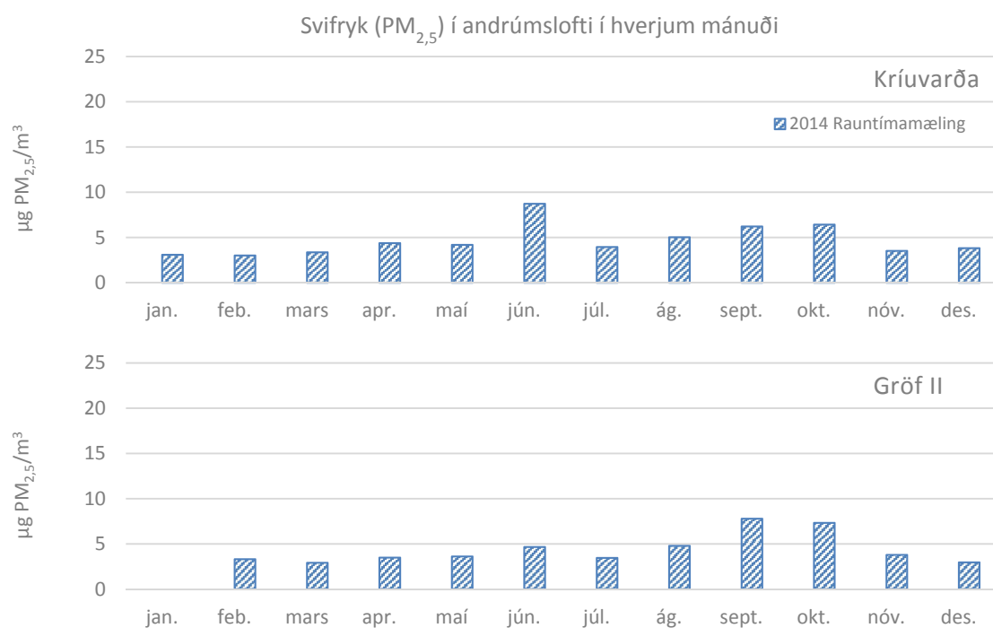
Mynd 4.19: Meðalstyrkur svifryks ( PM_{2,5} ) í hverjum mánuði að Kríuvörðu og Gröf II árið 2014
