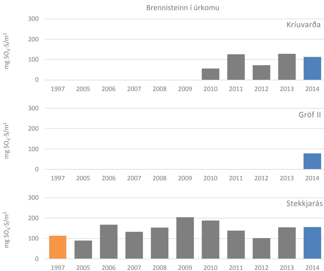
Mynd 4.24: Meðalstyrkur brennisteins í úrkomu að Kríuvörðu, Gröf II og Stekkjarási á vöktunartímabilinu
