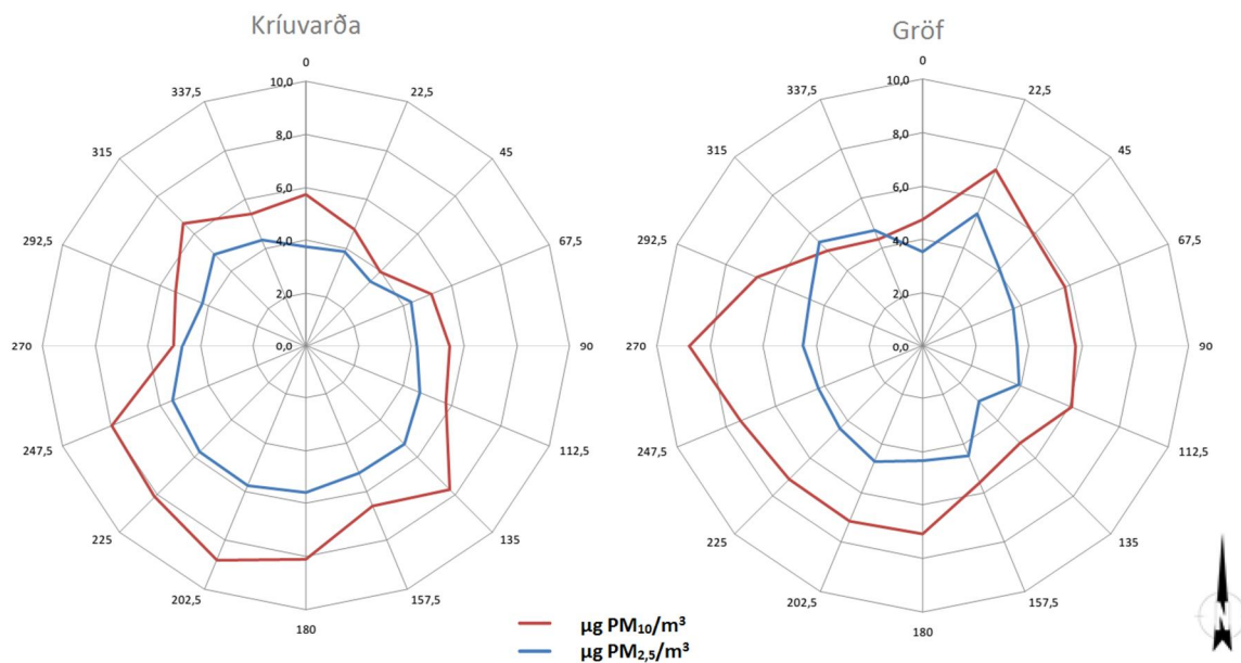
Mynd 4.20: Styrkur svifryks ( \mu\text{g PM}/\text{m}^3 ) eftir vindáttum að Kríuvörðu og Gröf II árið 2014
