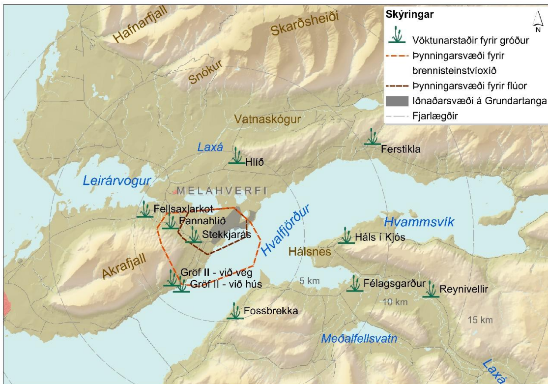
Mynd 8.1: Vöktunarstaðir fyrir gróður í Hvalfirði árið 2014
