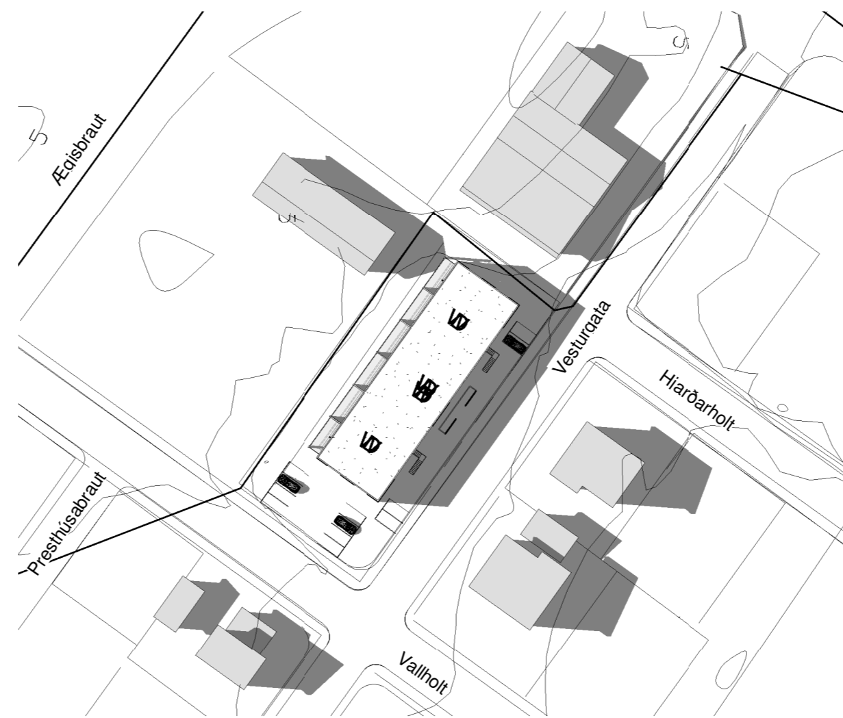
5 Grunnmynd svæðis sumarsólstöður kl 19,00 1 : 1000
