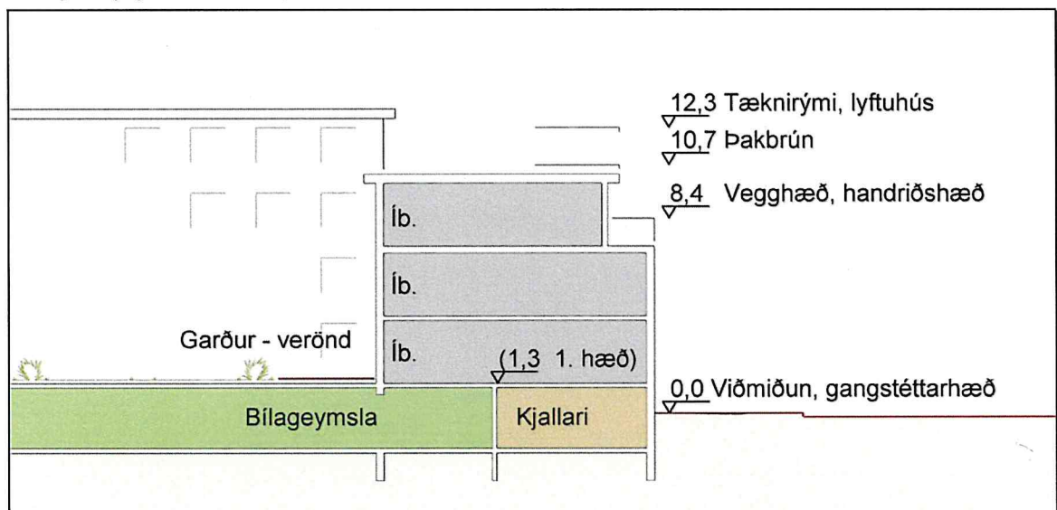
21. mynd Þriggja hæða hús við Dalbraut, Dalbraut 6. Þriggja hæða álma Dalbrautar 8.
