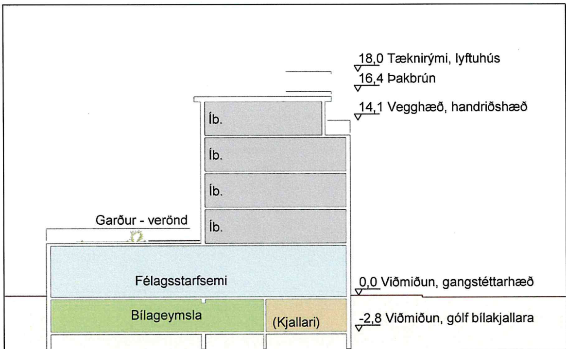
25. mynd Hús með félagsstarfsemi á fyrstu hæð. Dalbraut 4. Útfærsla með aukinni lofthæð og alniðurgrafinni bílageymslu.
