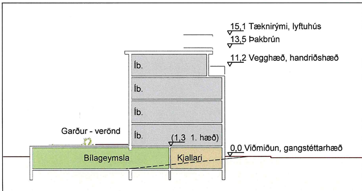
20. mynd Fjögurra hæða hús, Dalbraut 6.
