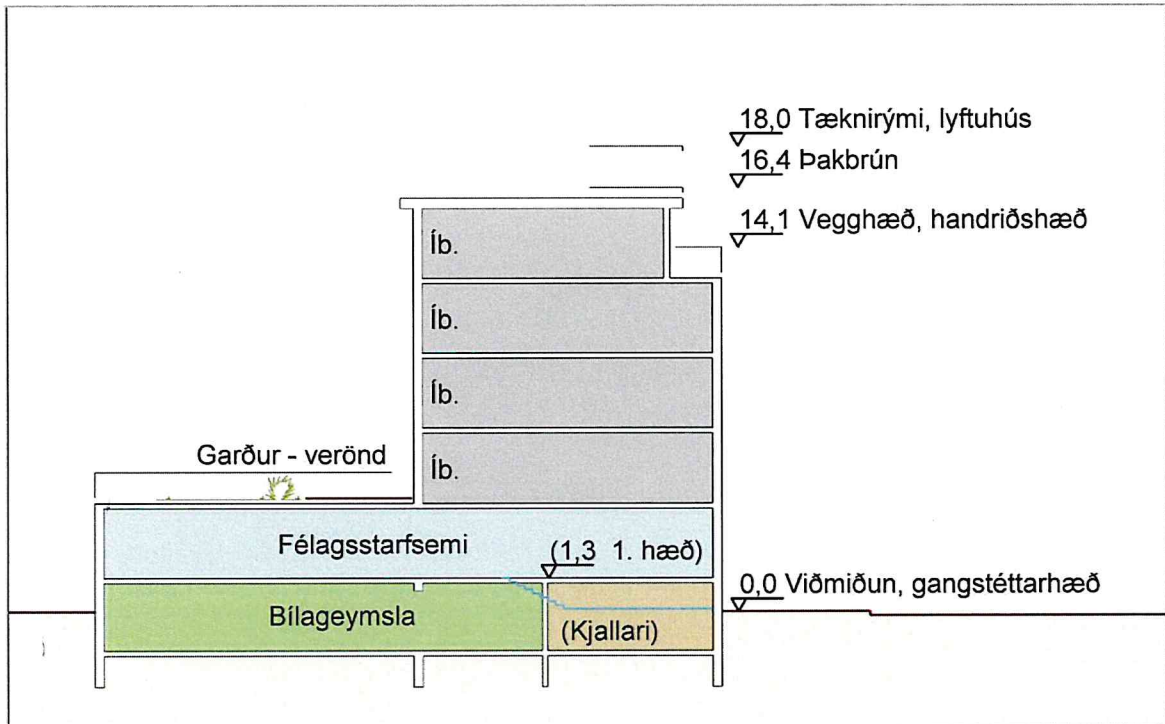
24. mynd Hús með félagsstarfsemi á fyrstu hæð. Dalbraut 4.
