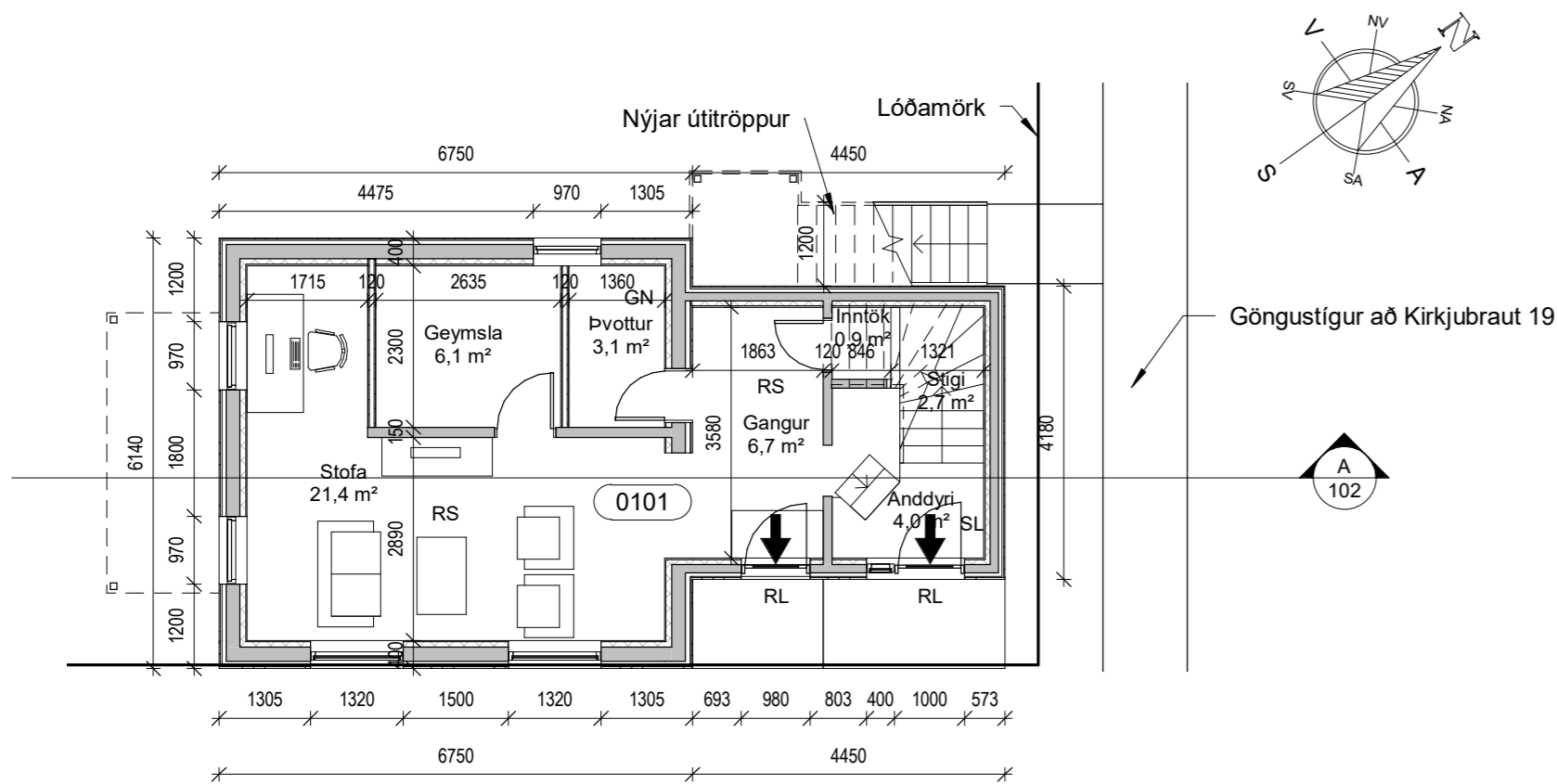
1. hæð 1 : 100
