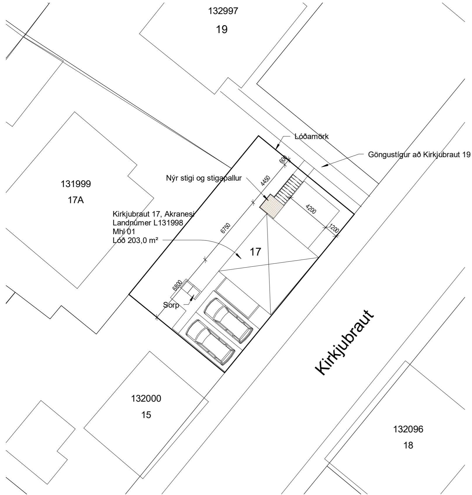
Afstöðumynd 1 : 200
