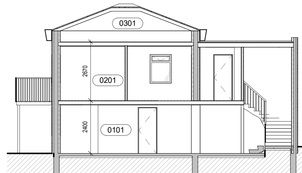
Snið A 1 : 100
