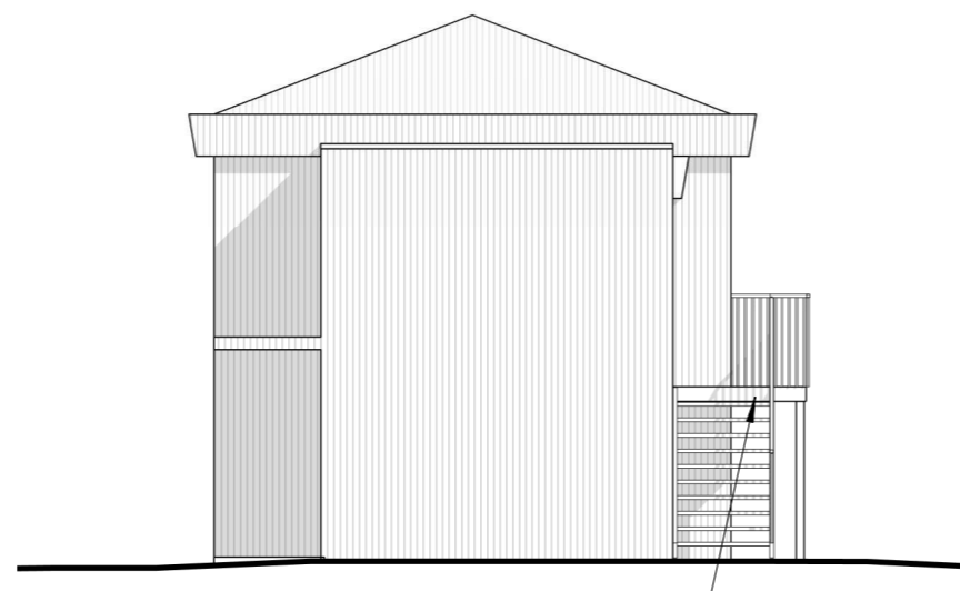
Norðausturhlið 1 : 100
