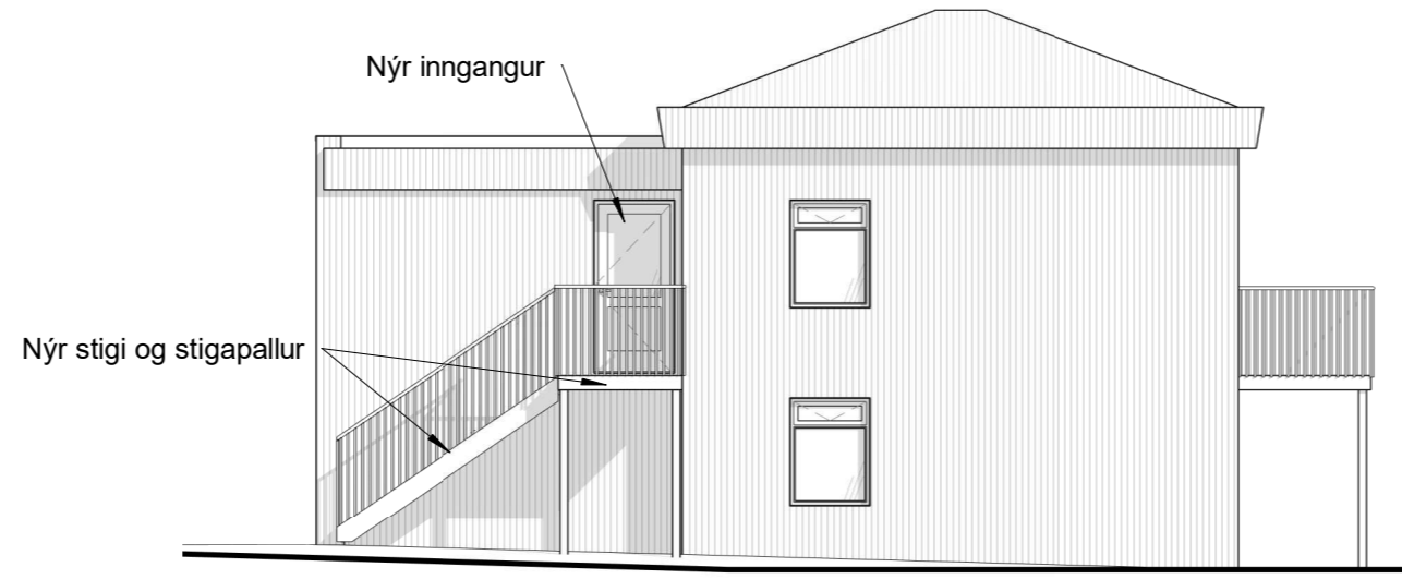
Norðvesturhlið 1 : 100
