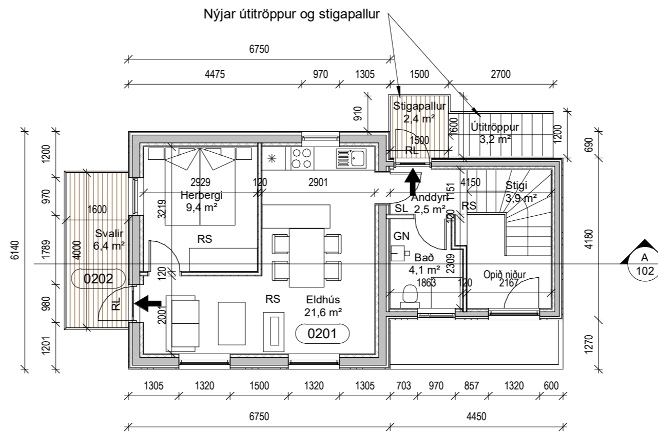
2. hæð 1 : 100
