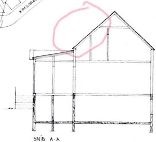
SNIB A-A
